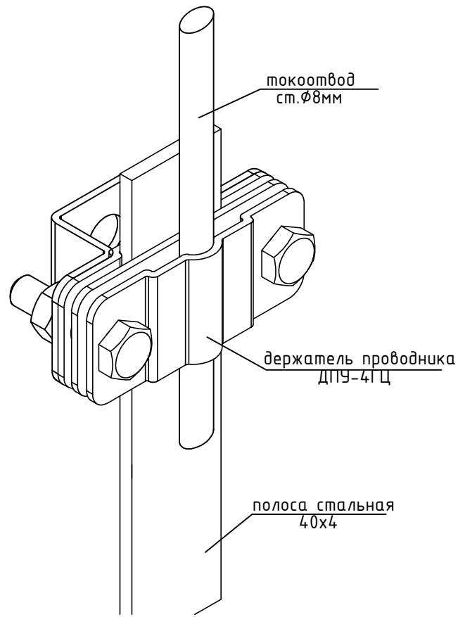
Узел соединения токопровода и полосы заземления на фасаде на отм. +0,700
