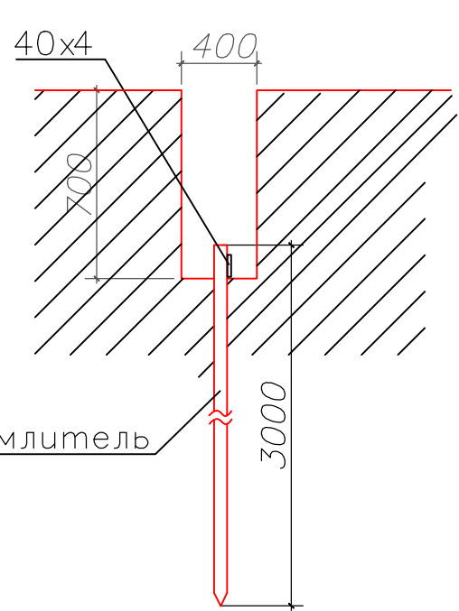
Траншея Т-3
