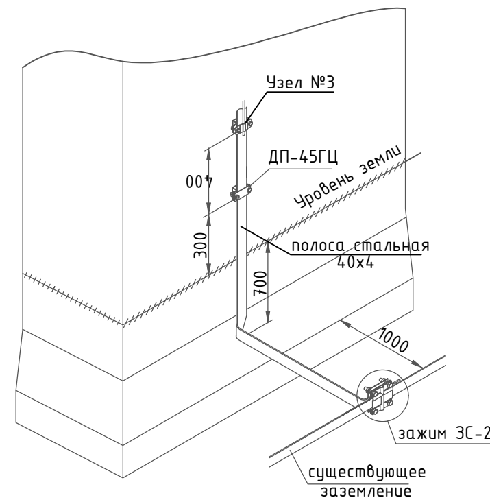
Узел соединения токопровода и полосы заземления в земле на отм. -0,700
